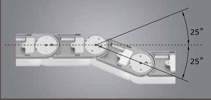
Modül mafsıl hareketi / Rotating pivot joints
